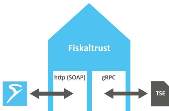
Abbildung 14: Kommunikation über http(SOAP) und gRPC
