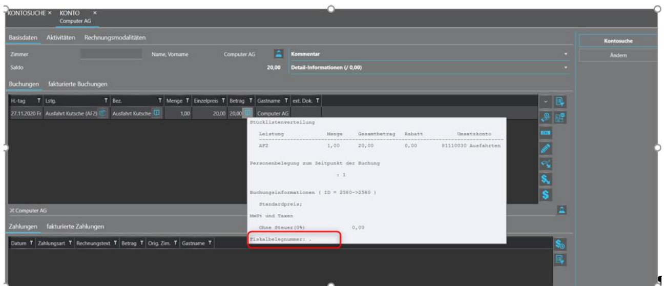
Abbildung 86: Buchung Tooltip fehlende Belegnummer Flex-Client
