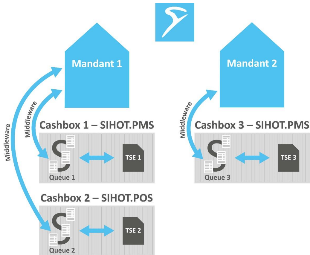
Abbildung 2: Kommunikationsmodell in einer Multi-Mandant Umgebung
